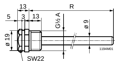
ALT-SB..., ALT-SS...
