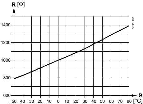
Рабочая характеристика:
